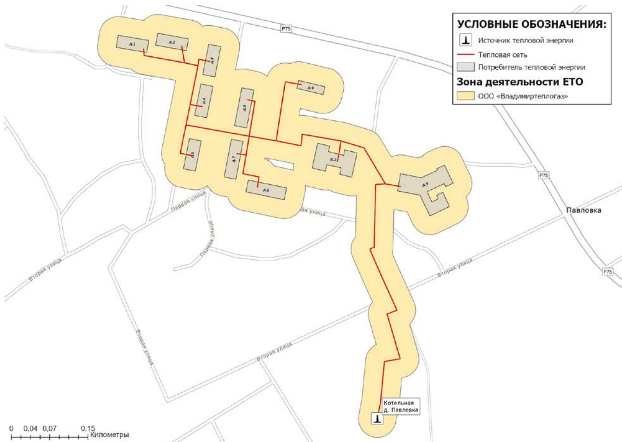
Рисунок 15.5.5 - Границы зоны деятельности единой теплоснабжающей организации на территории
