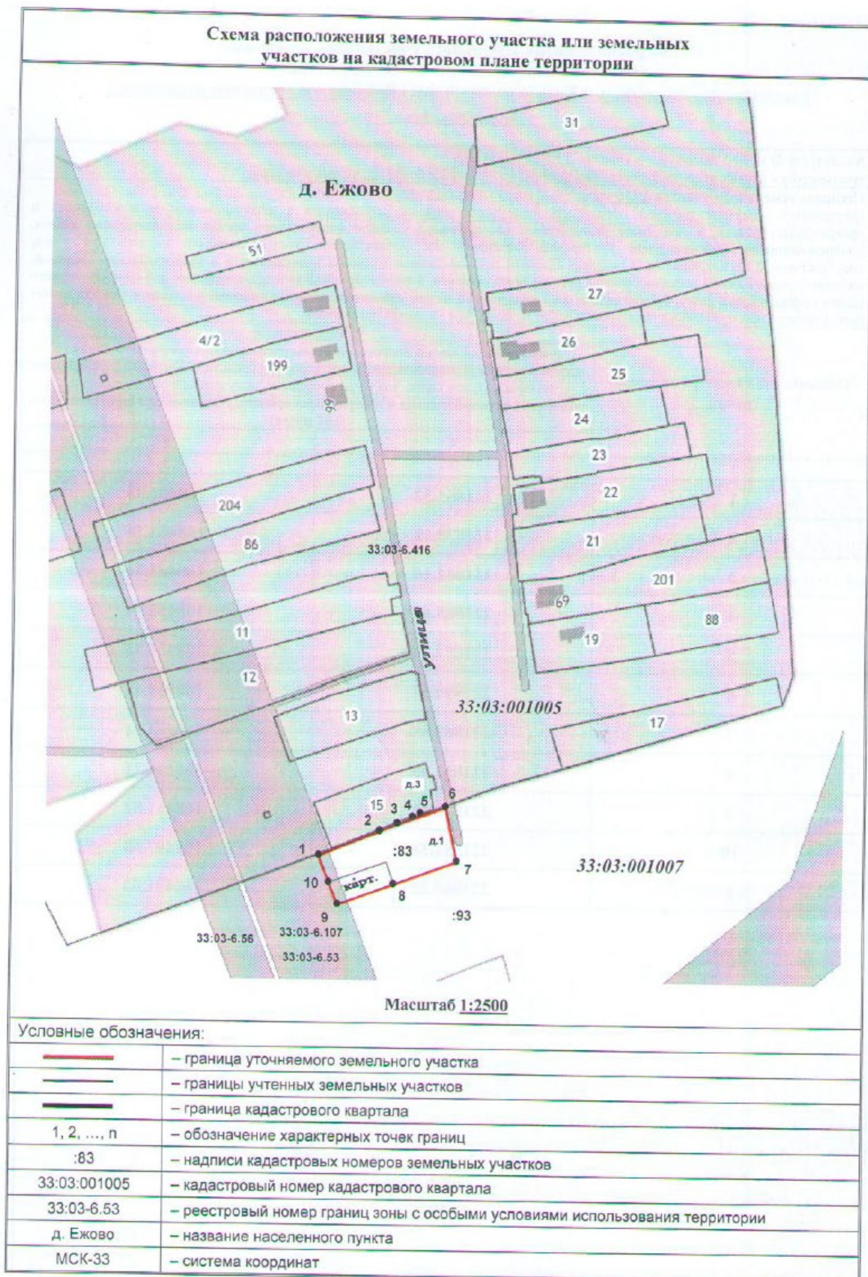
Рис. 1 Схема расположения земельного участка
